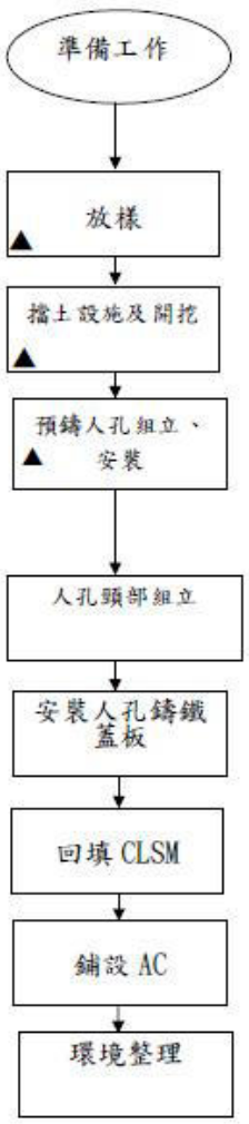
施工作業流程圖
